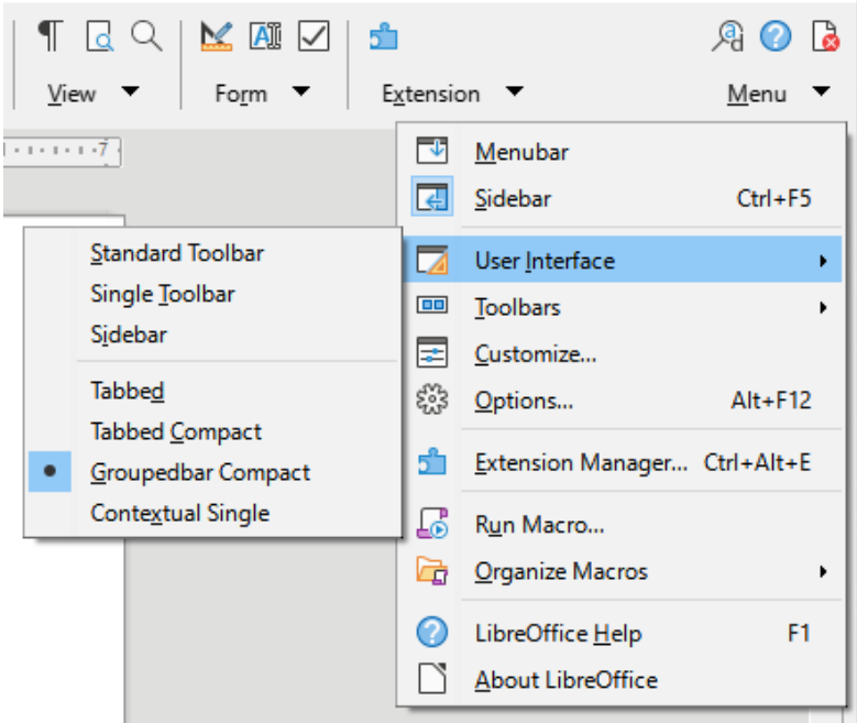
Figure 501: Groupedbar menu
