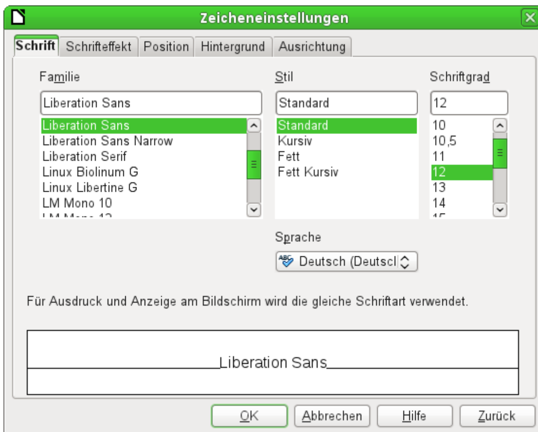
Abbildung 49: Schrift - Zeicheneinstellungen
