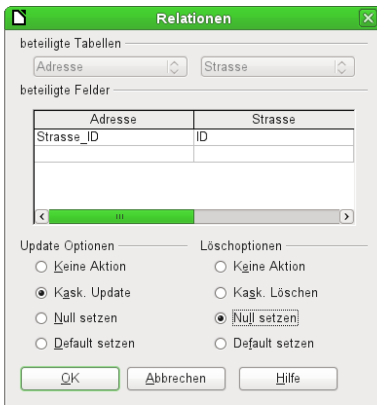
Abbildung 13: Dialog «Relationen»
