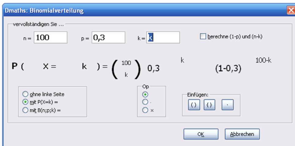
Abbildung 35: Dialog Binomialverteilung
