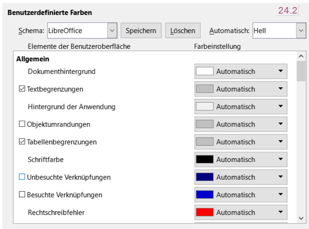
Abbildung 3: Ein- und Ausblenden von Text-, Objekt- und Tabellengrenzen und Farbgebung
