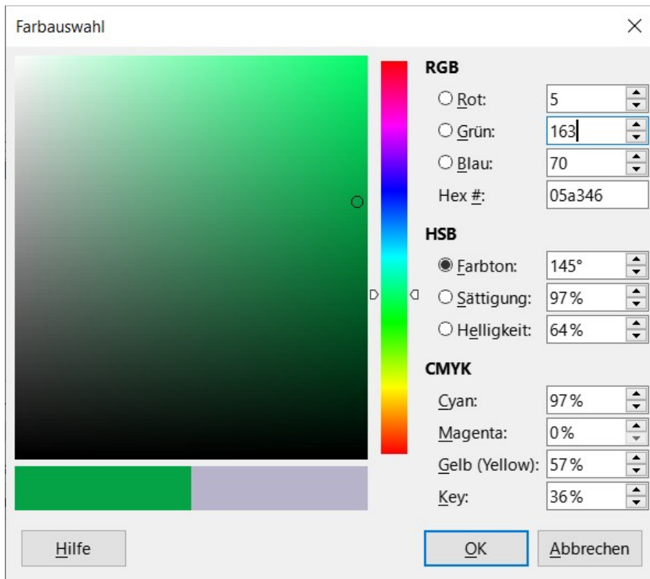
Abbildung 30: Dialog „Farbauswahl“
