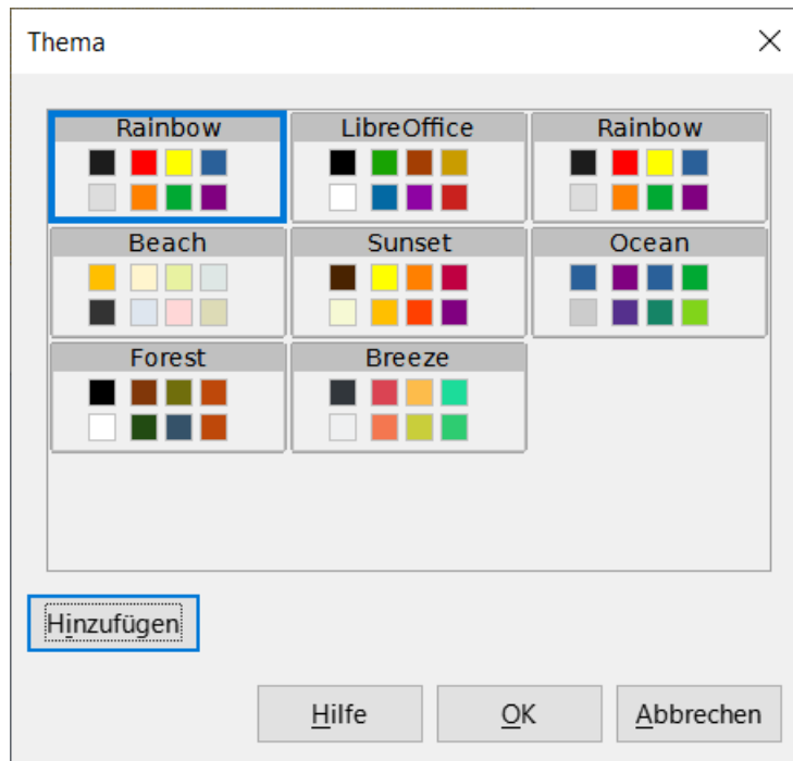
Abbildung 31: Dialog „Thema“
