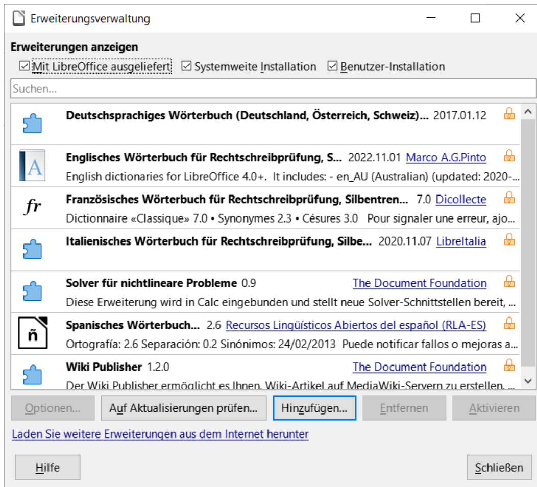
Abbildung 28: Dialog „Erweiterungsverwaltung“
