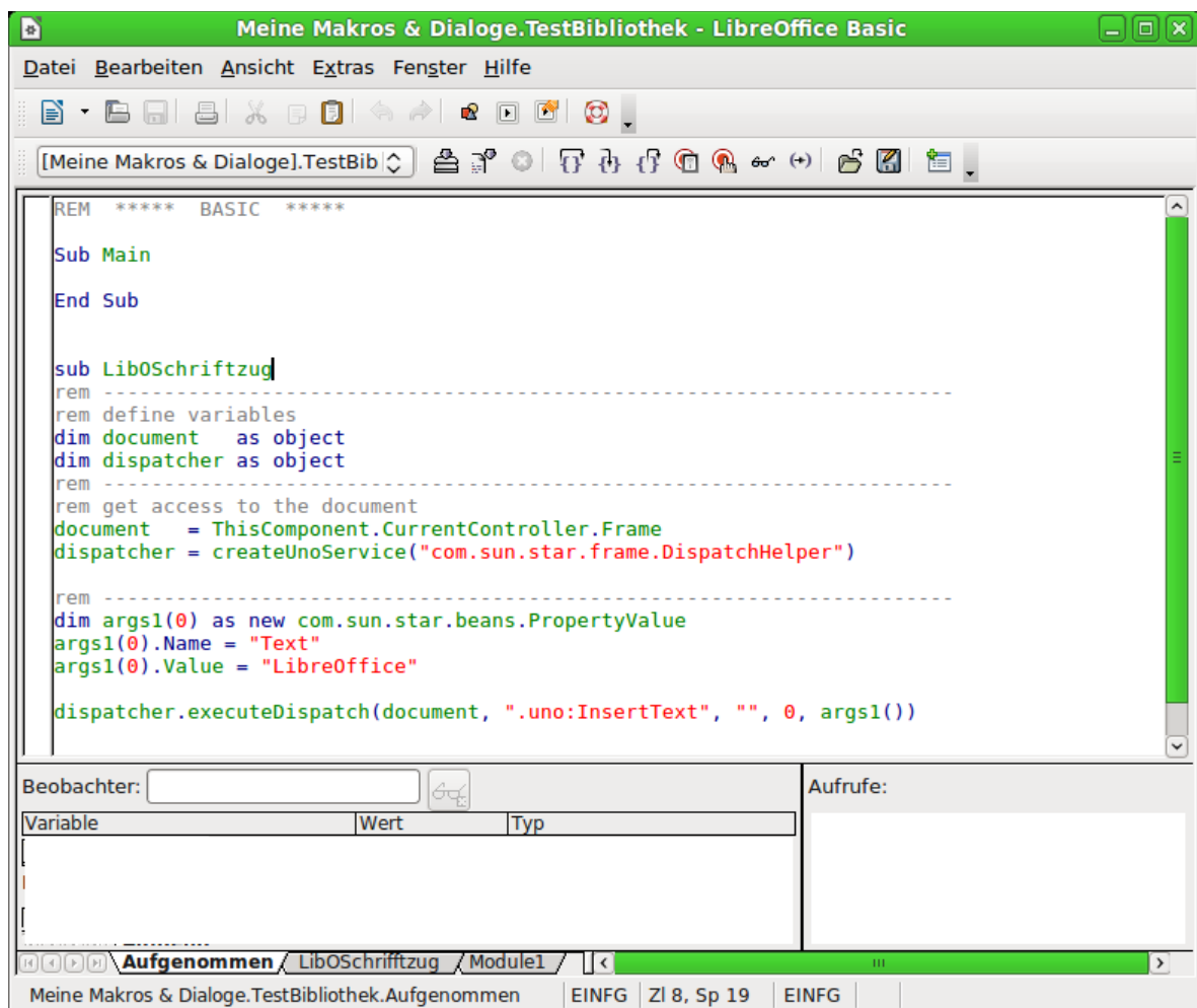
Abbildung 7: IDE
