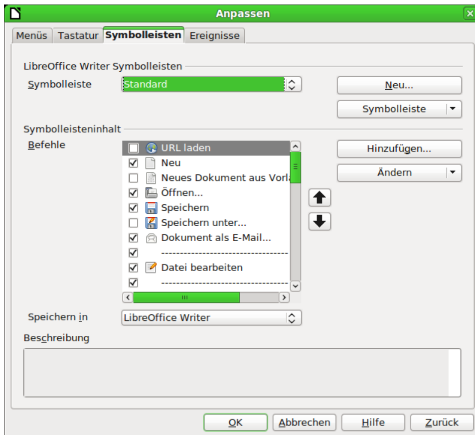
Abbildung 15: Symbolleisten anpassen
