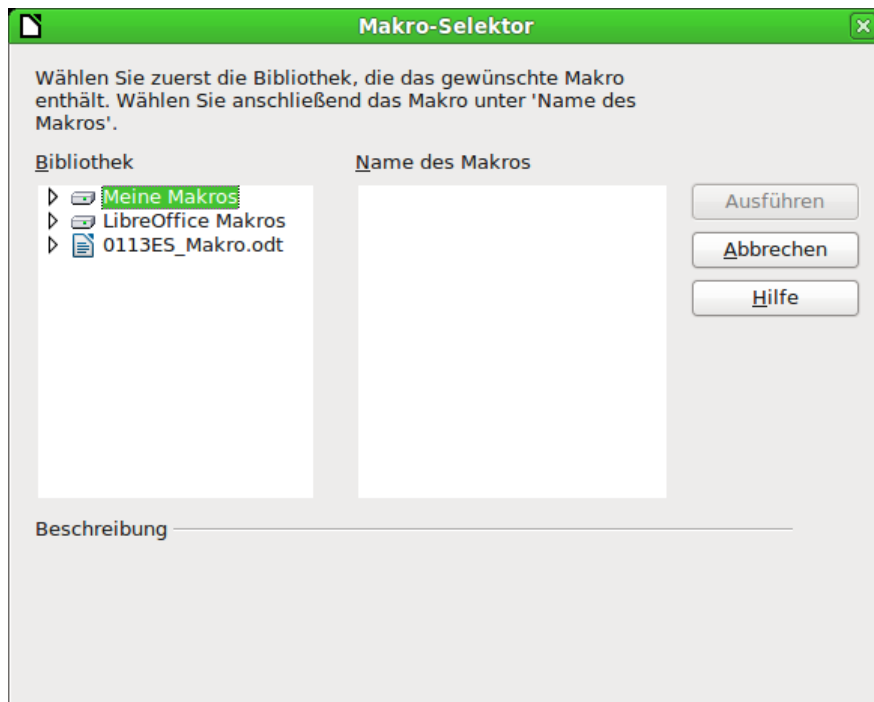
Abbildung 14: Makro Selektor
