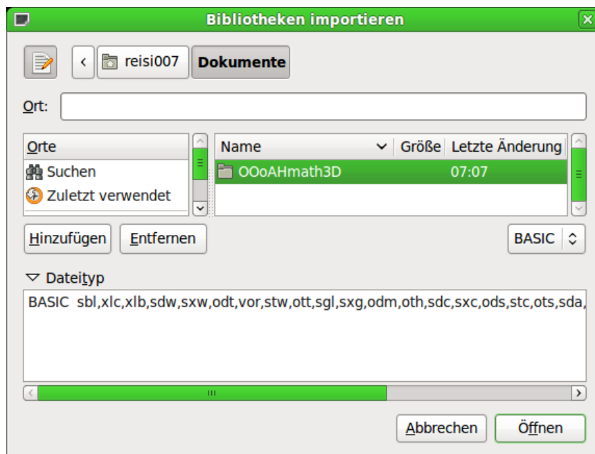
Abbildung 11: Bibliothek importieren 1
