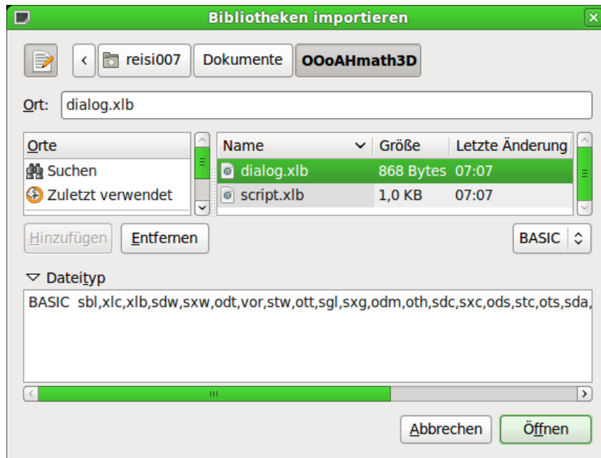
Abbildung 12: Bibliothek importieren 2
