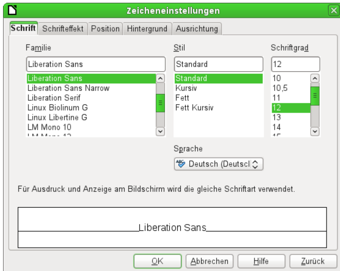
Abbildung 2: Schrift - Zeicheneinstellungen
