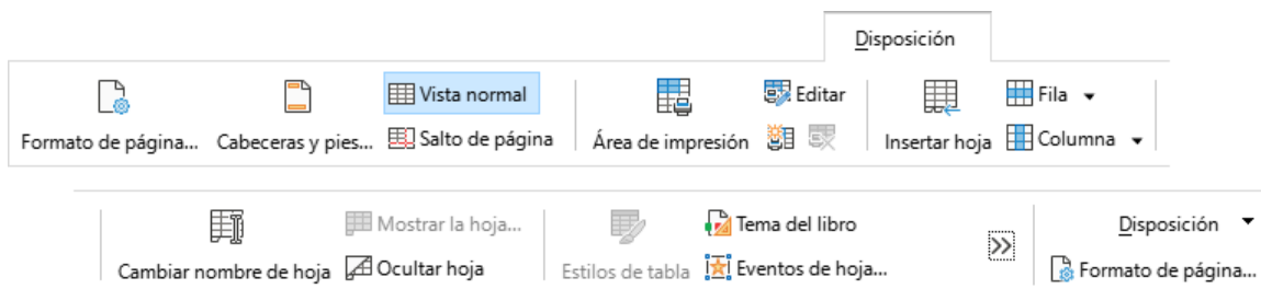
Figura 548: Pestaña Disposición.
