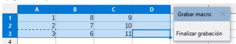
Figura 461: Grabar macro
