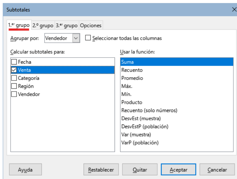
Figura 339: Diálogo Subtotales
