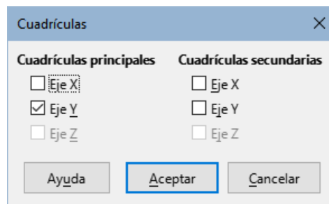
Figura 98: Diálogo Cuadrículas
