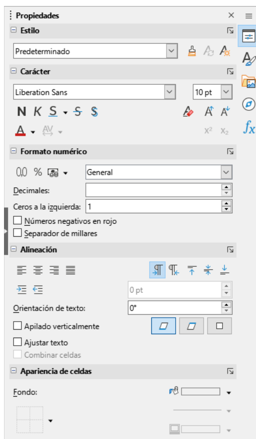
Figura 8: Barra lateral
