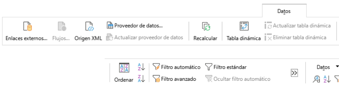
Figura 551: Pestaña Datos.
