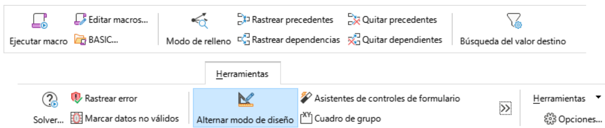
Figura 561: Pestaña Herramientas .
