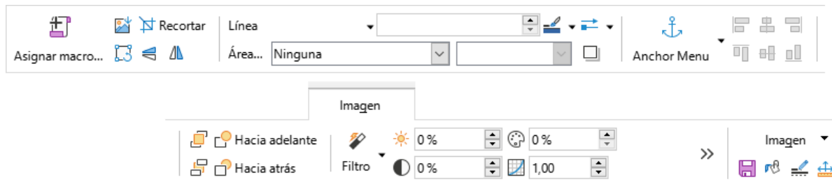
Figura 569: Pestaña Imagen.
