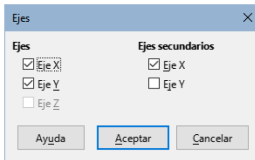
Figura 82: Diálogo Ejes
