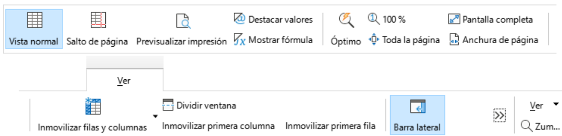
Figura 557: Pestaña Ver.
