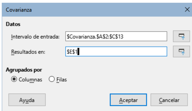
Figura 373: Diálogo Covarianza
