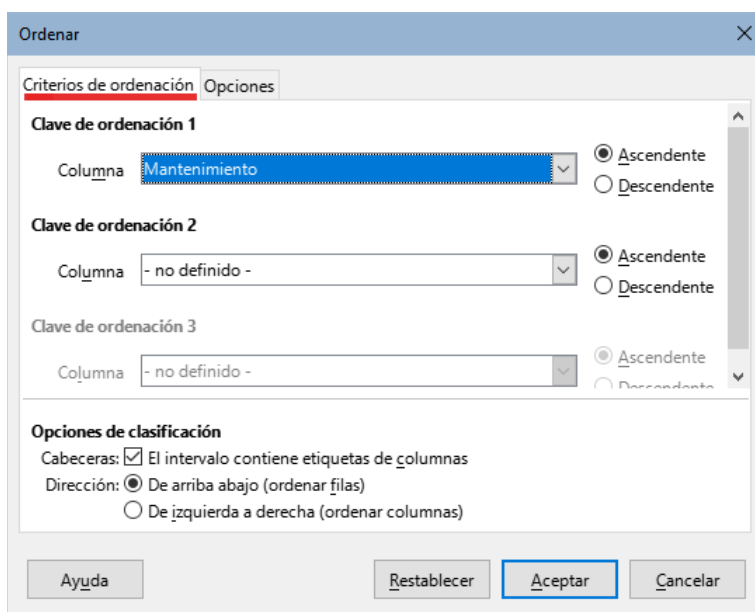
Figura 495: Diálogo Ordenar.
