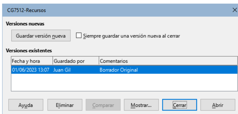
Figura 457: Diálogo Versiones
