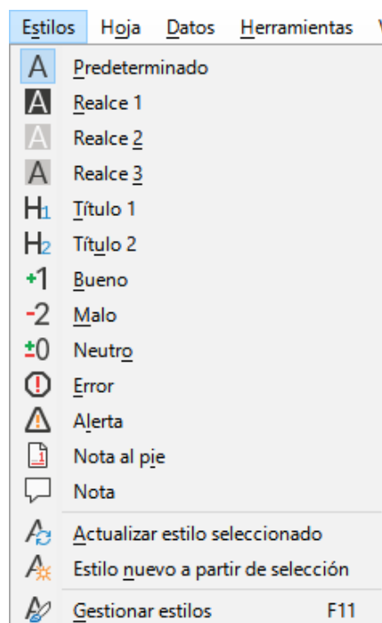
Figura 179: Menú Estilos
