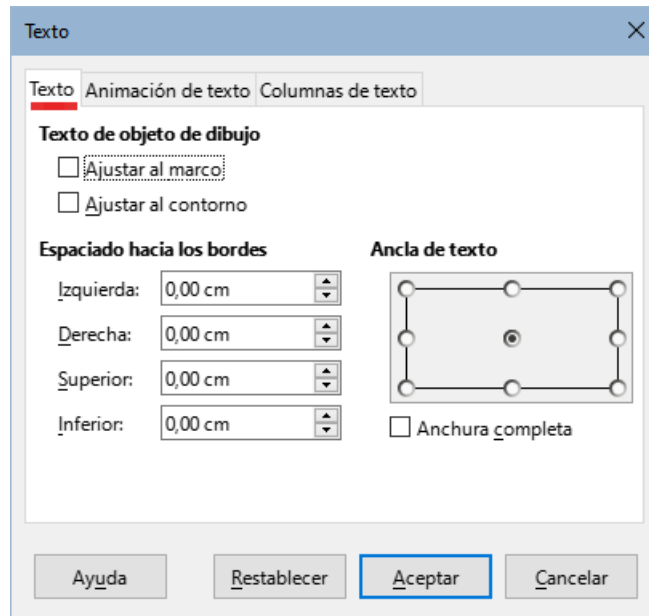
Figura 210: Diálogo Texto
