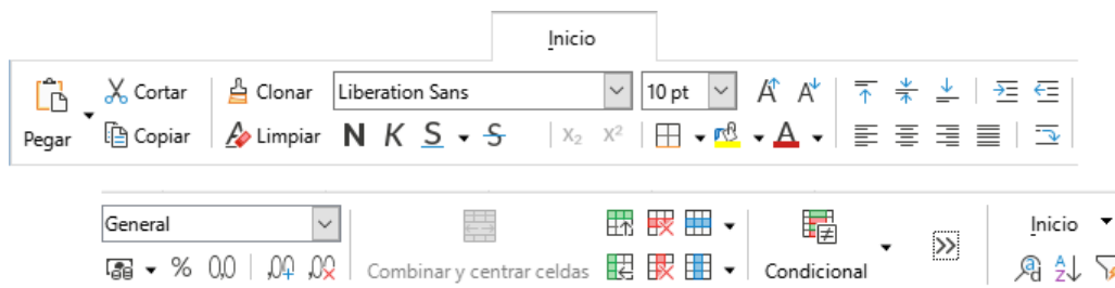
Figura 542: Pestaña Inicio.
