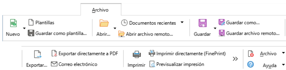
Figura 539: Pestaña Archivo.
