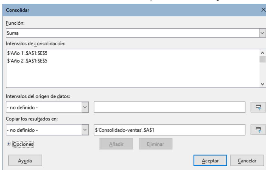
Figura 331: Diálogo Consolidar
