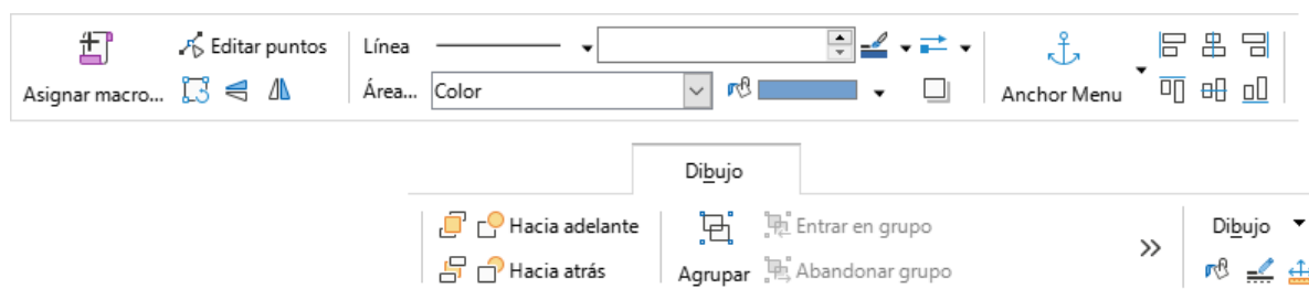
Figura 564: Pestaña Dibujo .
