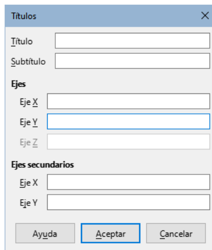
Figura 69: Diálogo Títulos
