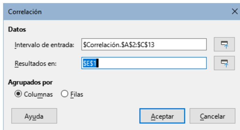
Figura 371: Diálogo Correlación
