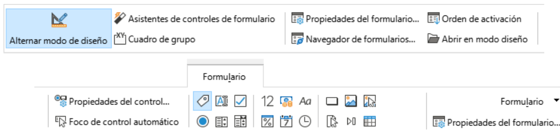
Figura 567: Pestaña Formulario .
