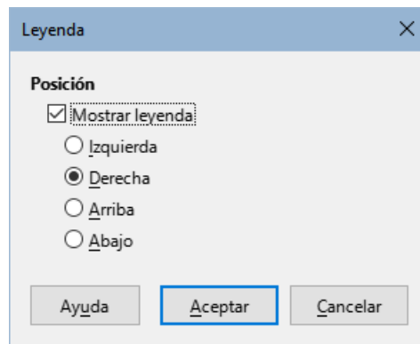
Figura 72: Diálogo Leyenda
