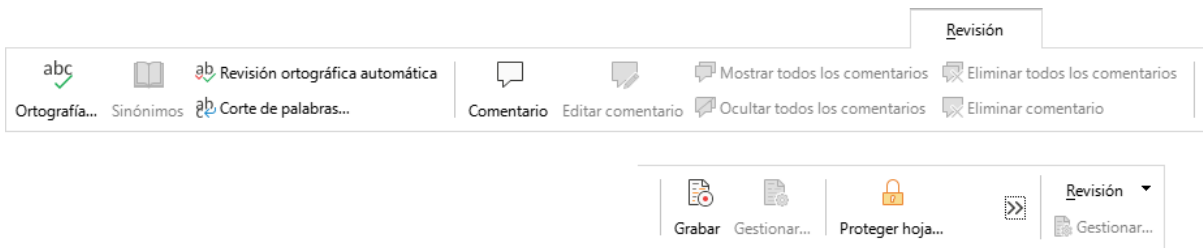
Figura 554: Pestaña Revisión.
