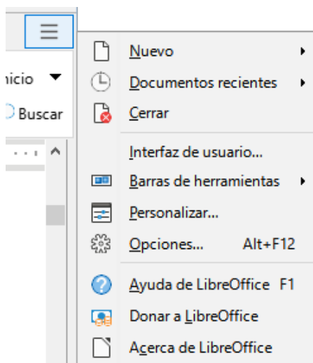
Figura 538: Menú rápido.
