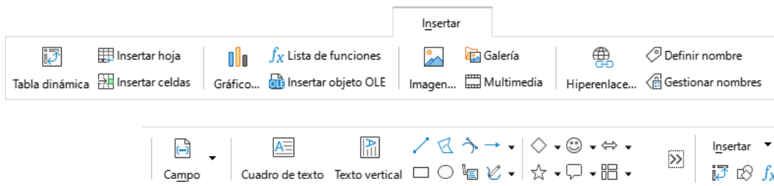
Figura 545: Pestaña Insertar.
