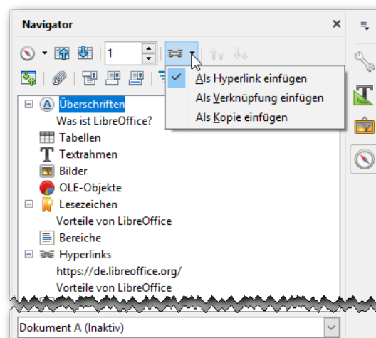
Abbildung 1: Hyperlinks mit dem Navigator einfügen
