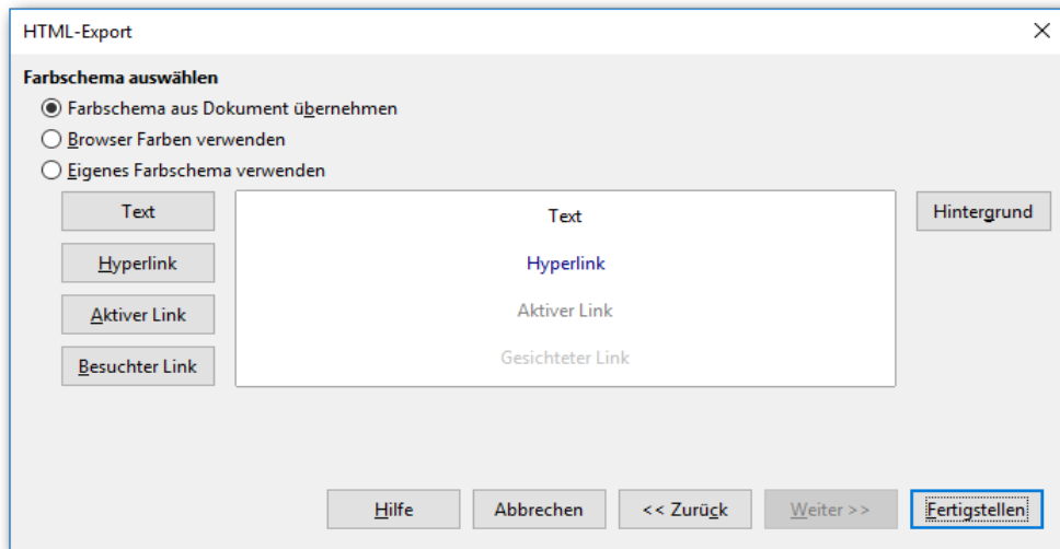
Abbildung 9: HTML-Export - Farbschema
