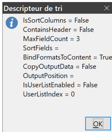
Figure 13 : Informations contenues dans un descripteur de tri.
