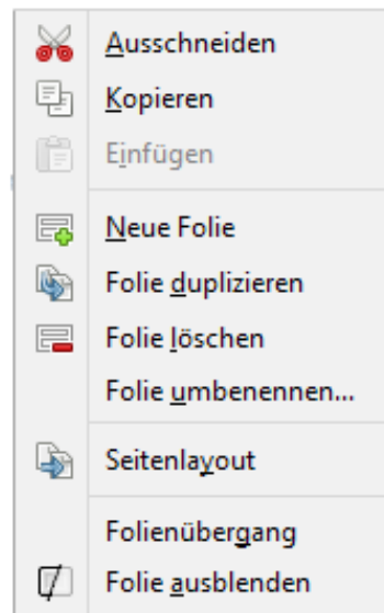
Abb. 7 Kontextmenü
