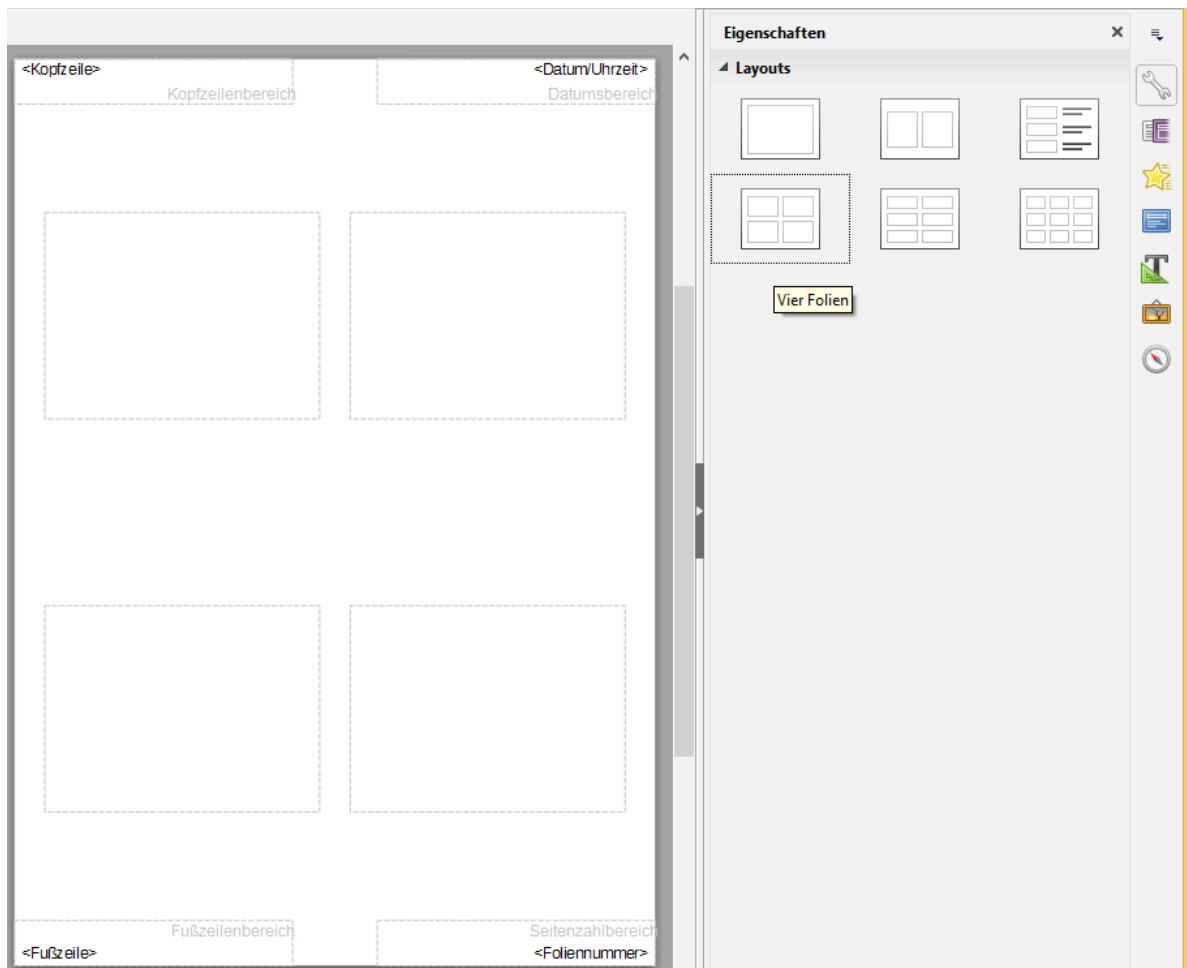
Abb. 6: Handzettel-Layout-Auswahl
