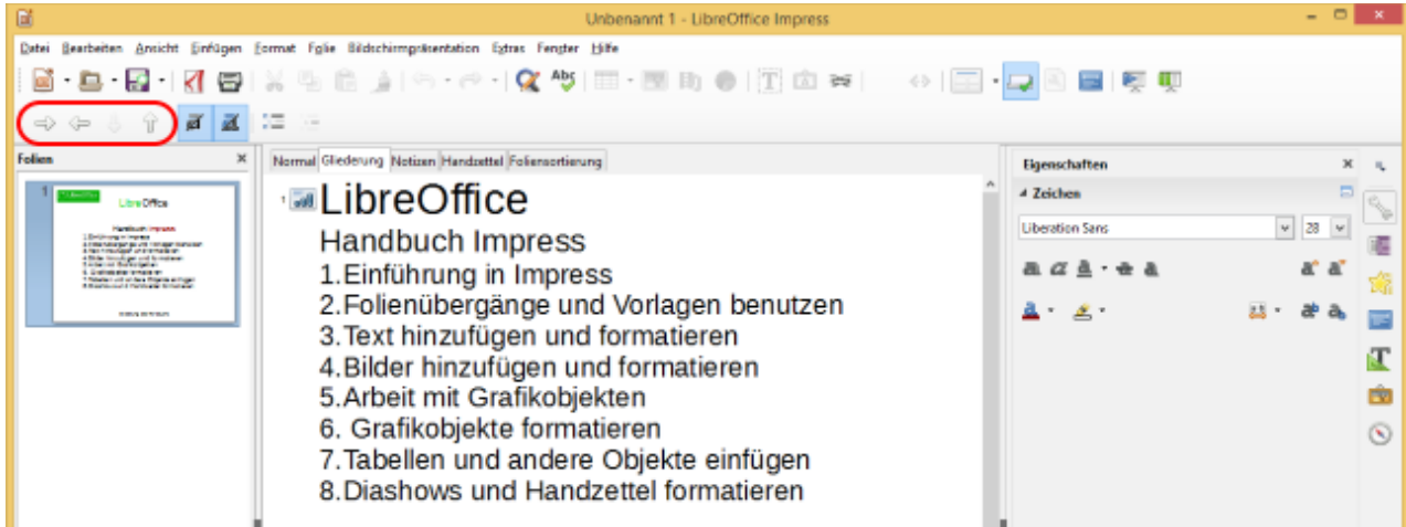
Abb. 4 Ansicht Gliederung
