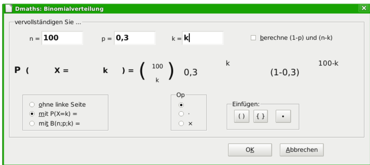
Abbildung 8: Dialog Binomialverteilung
