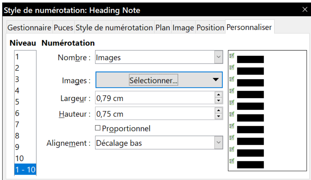
Figure 21 : Paramétrer la taille et l'alignement de l'image qui servira de puce.
