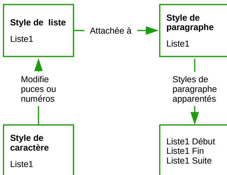
Figure 8 : Donnez des noms semblables aux styles apparentés pour retrouver plus facilement ceux dont vous avez besoin.
