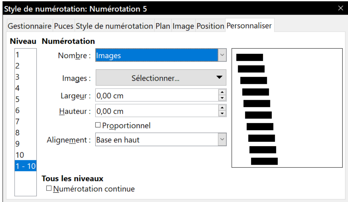
Figure 17 : Les champs qui permettent de paramétrer une image utilisée comme puce apparaissent quand vous avez choisi Images ou Images liées dans le champ Nombre .
