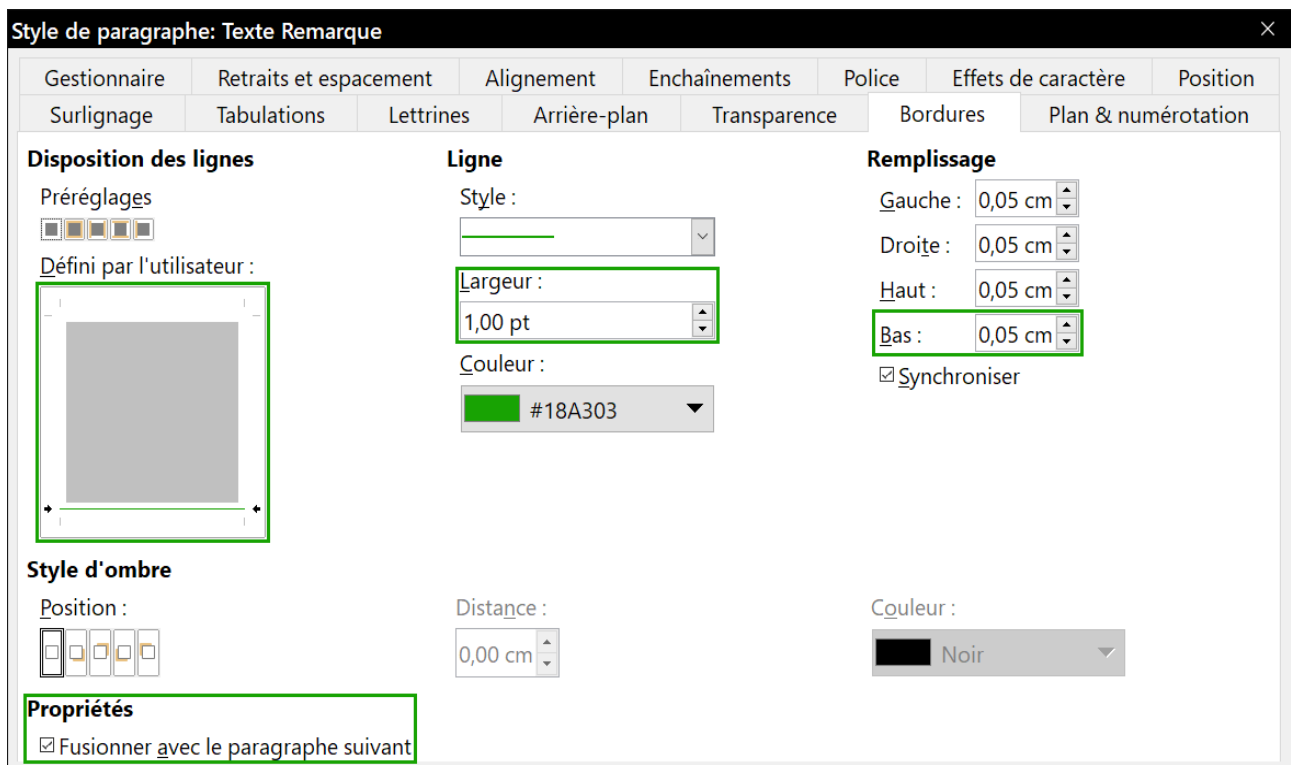
Figure 19 : Définir la bordure inférieure du corps de note
