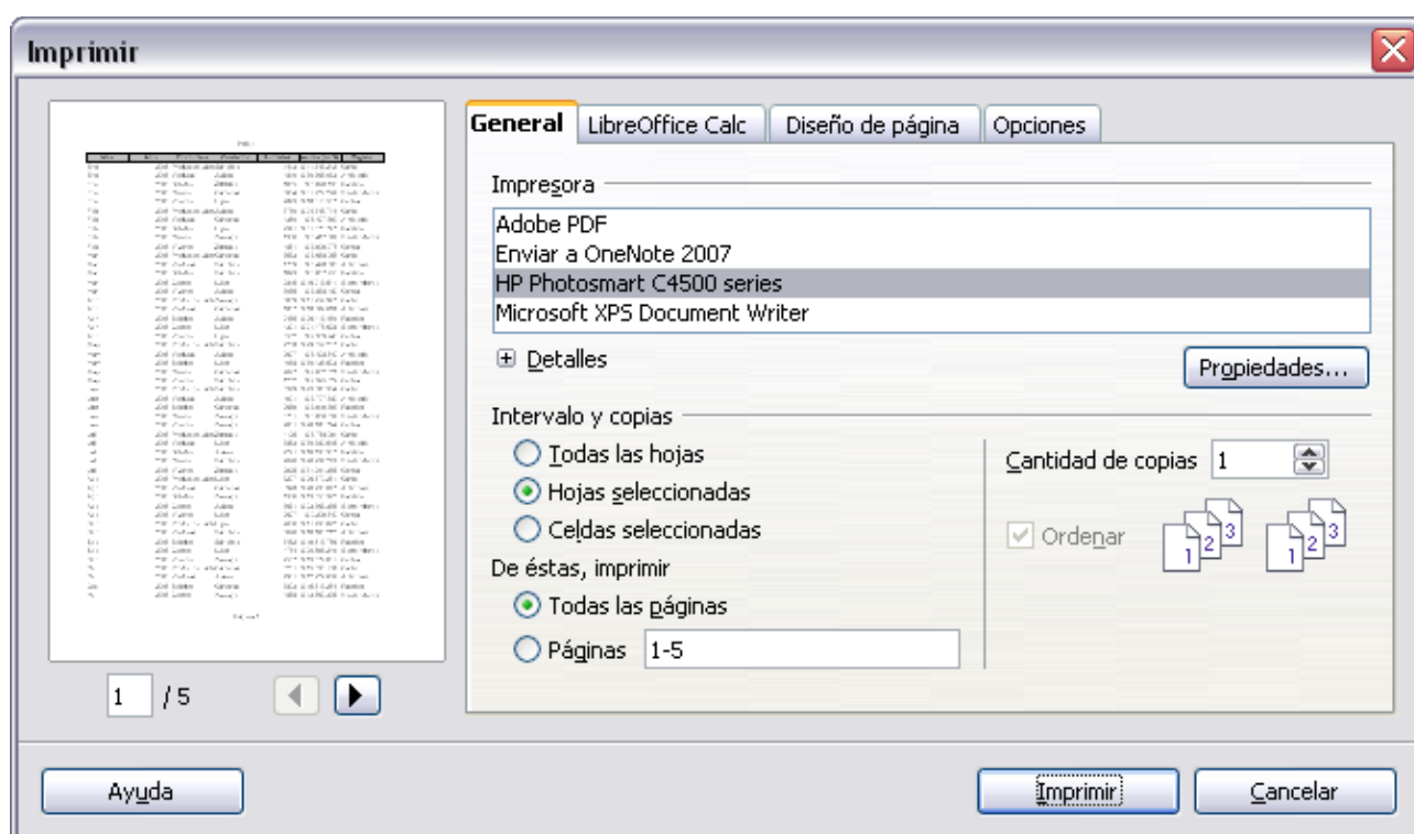
Figura 37: Diálogo Imprimir
