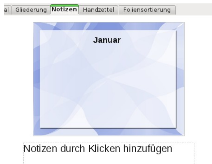
Abbildung 6: Ansicht Notizen
