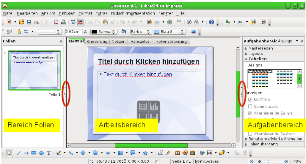
Abbildung 1: Das Impress-Hauptfenster
