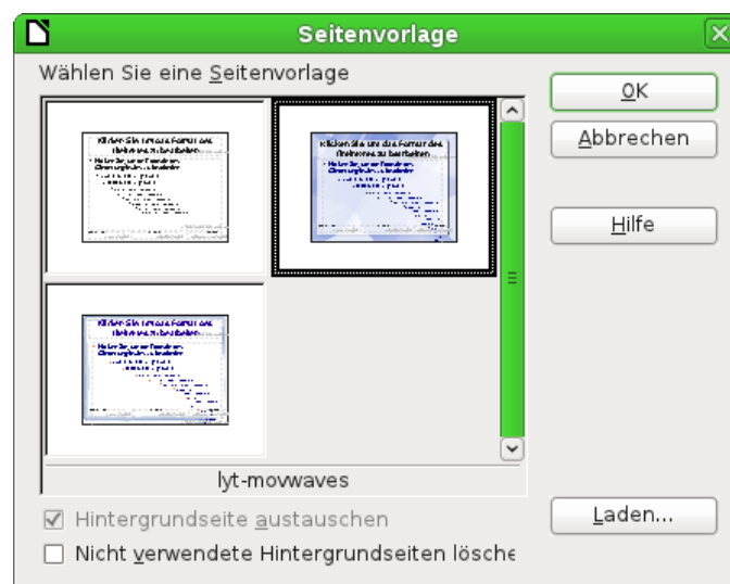
Abbildung 22: Dialog Seitenvorlage
