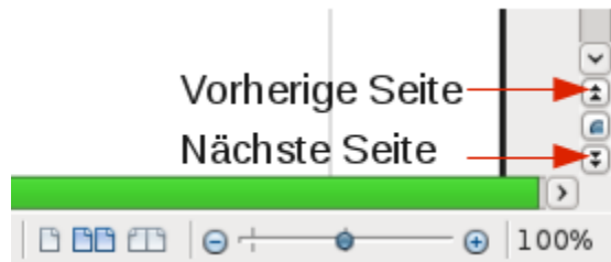
Abbildung 4: Navigation-Icons
