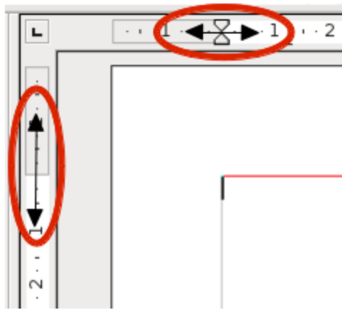
Abbildung 23: Seitenränder verändern
