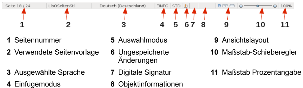
Abbildung 2: Statusleiste
