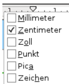
Abbildung 13: Maßeinheit wechseln
