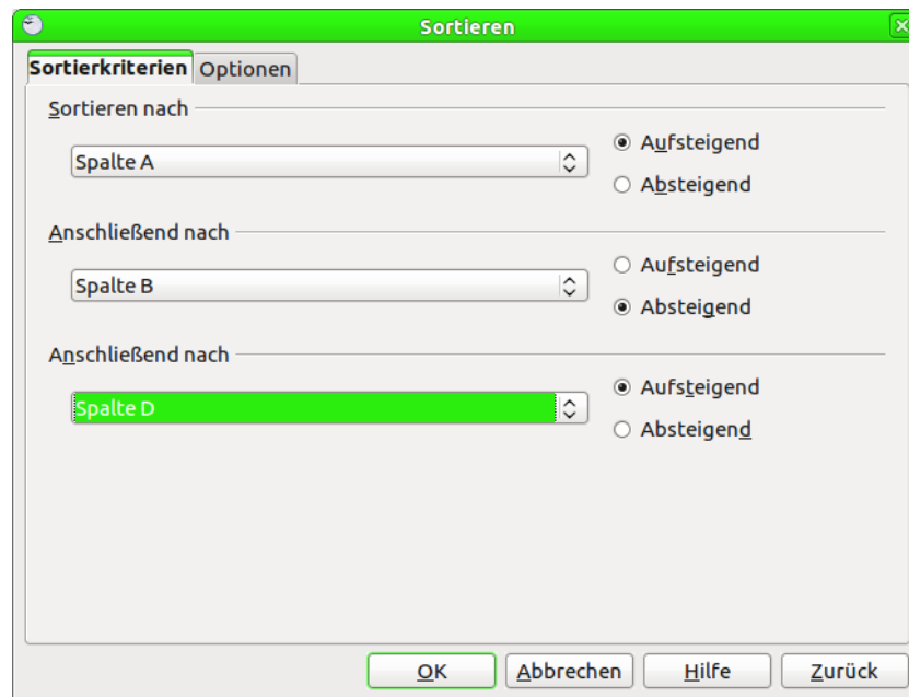
Abbildung 24: Sortierkriterien
