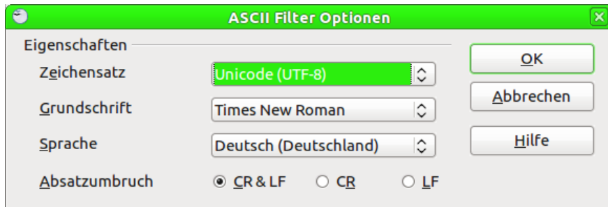
Abbildung 4: Dialog Textimport
