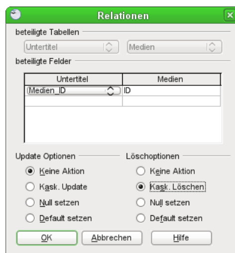
Abbildung 190: Abschnitt Update- und Löschoptionen
