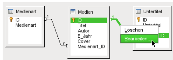
Abbildung 189: Bearbeitung der Relation zwischen "Medien" und "Untertitel"
