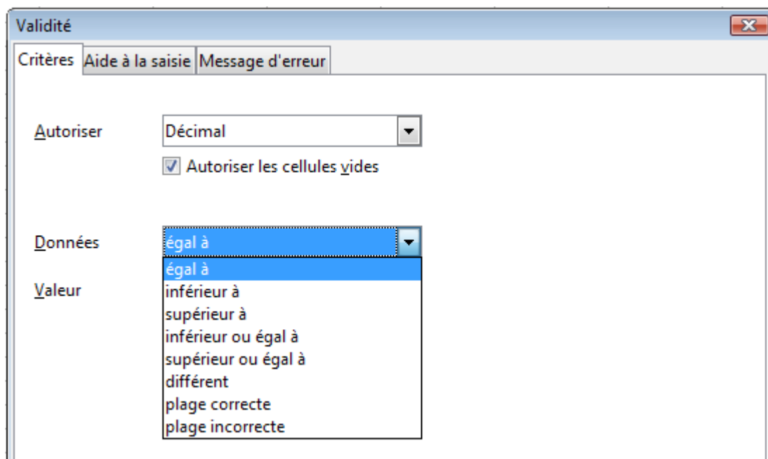
Figure 9 : Choix d'un test de validité ordinaire
