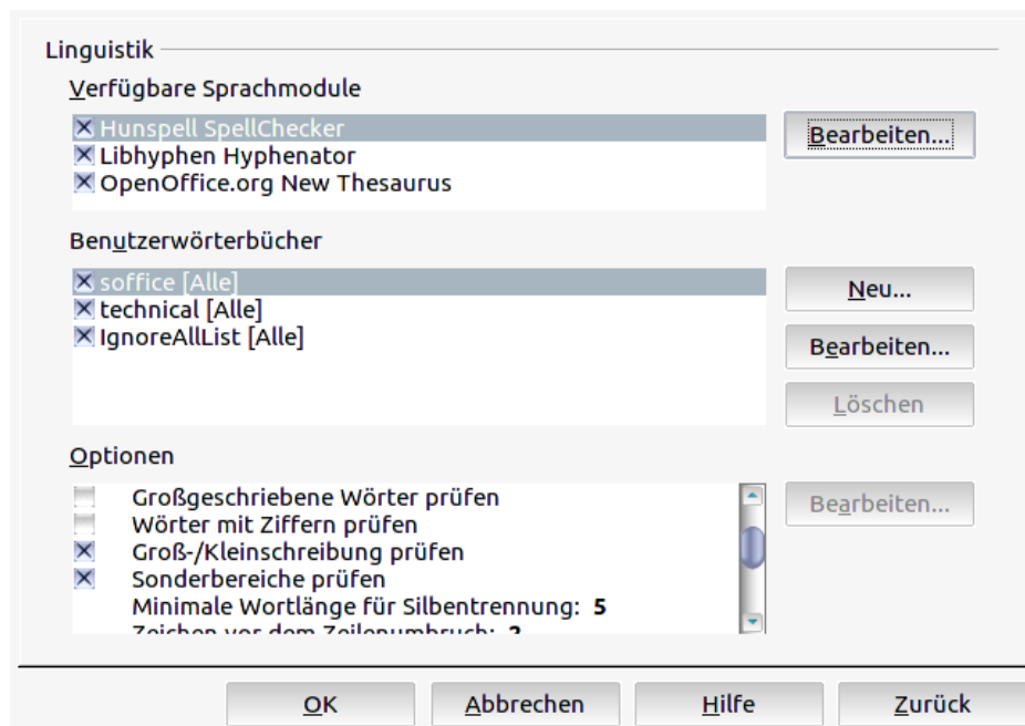
Abbildung 26: Spracheinstellungen - Linguistik
