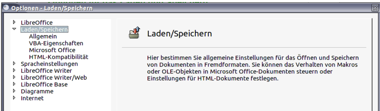
Abbildung 20: Laden/Speichern-Optionen
