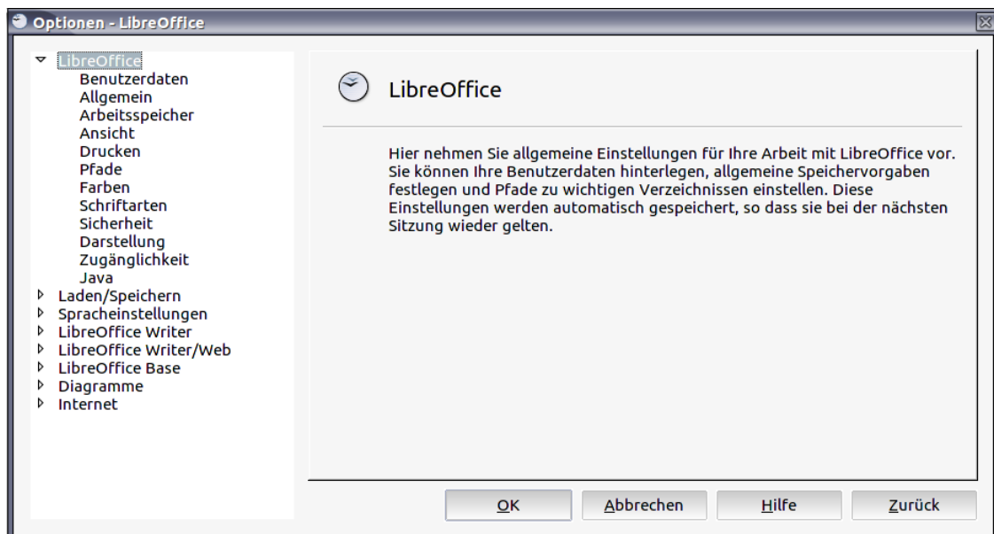
Abbildung 1: LibreOffice Optionen
