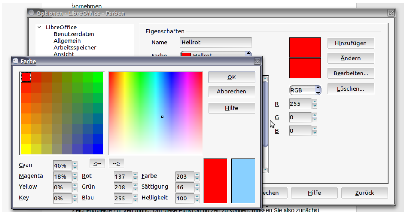
Abbildung 11: Farben bearbeiten
