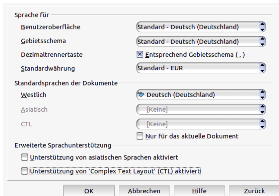
Abbildung 25: Spracheinstellungen
