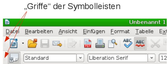
Abbildung 3: Angedockte Symbolleisten
