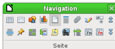
Abbildung 15: Navigationsleiste
