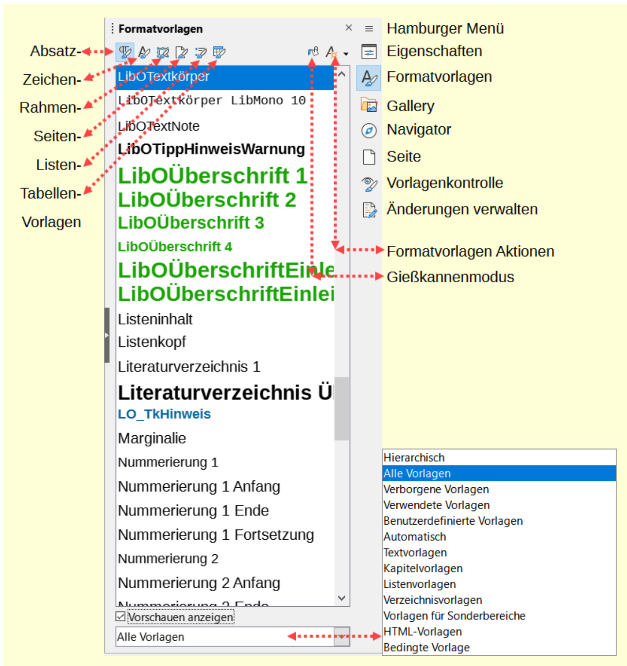
Abbildung 1: Seitenleiste "Formatvorlagen"
