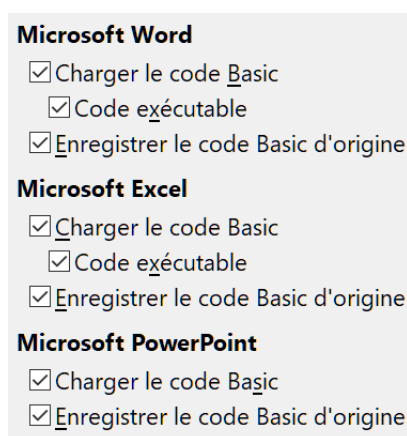
Figure 21 : Propriétés VBA
