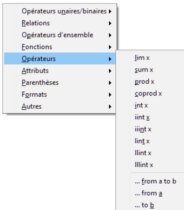
Figure 4 : Le menu contextuel de l'Éditeur de Formule
