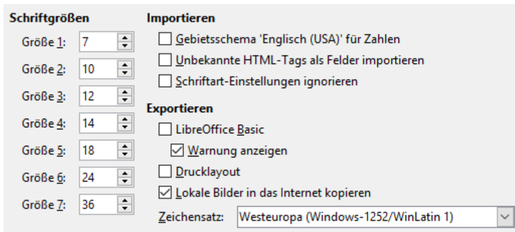
Abbildung 27: HTML-Kompatibilität
