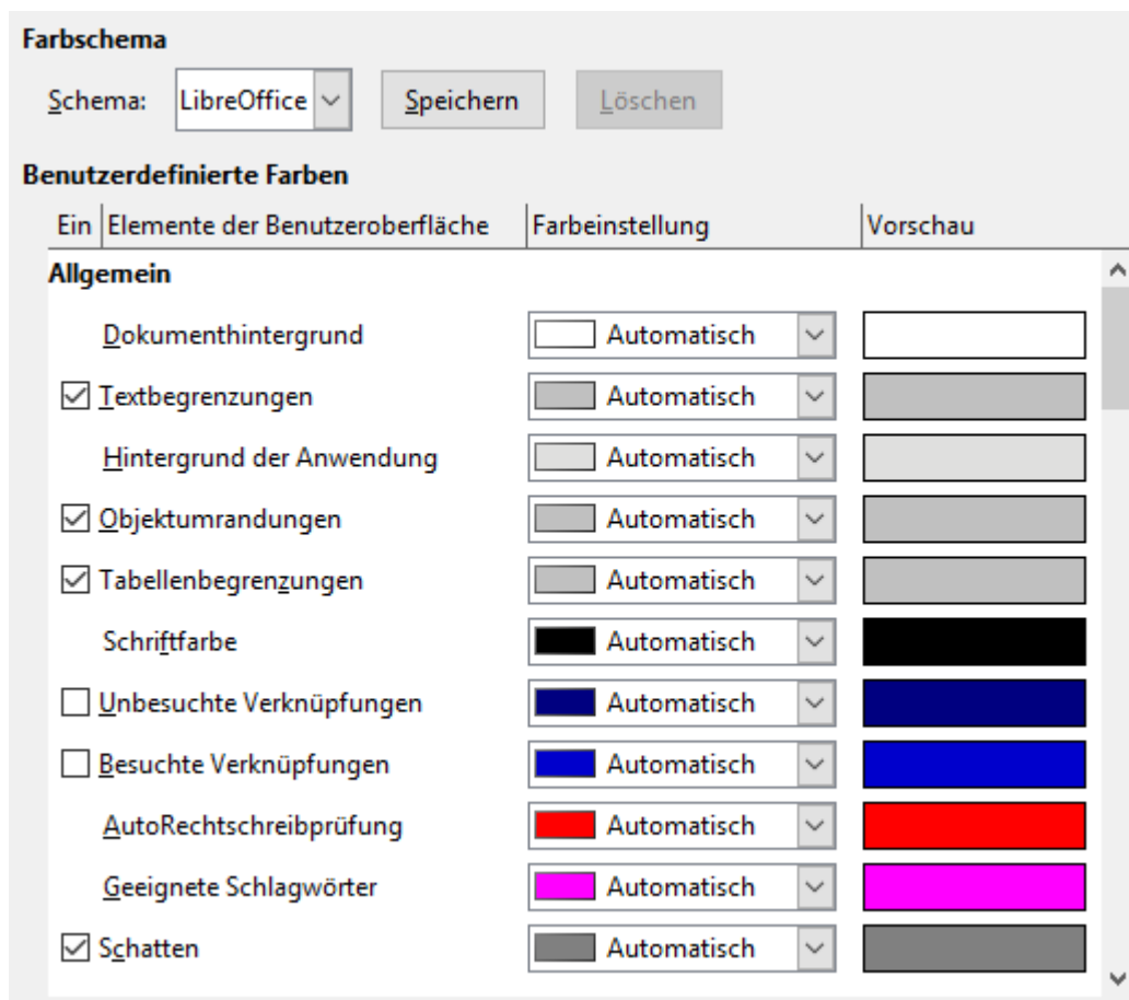
Abbildung 16: LibreOffice-Farbschema
