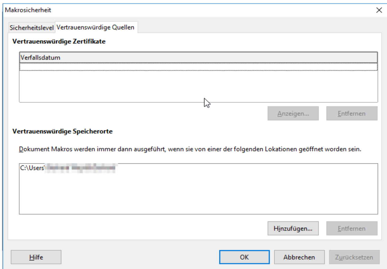
Abbildung 13: Vertrauenswürdige Quellen
