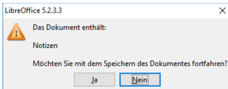
Abbildung 11: Sicherheitswarnung
