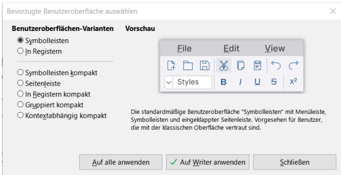
Abbildung 1: Benutzeroberflächen-Variante - Symbolleisten
