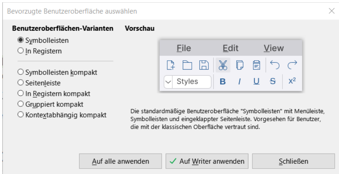
Abbildung 1: Benutzeroberflächen-Variante - Symbolleiste
