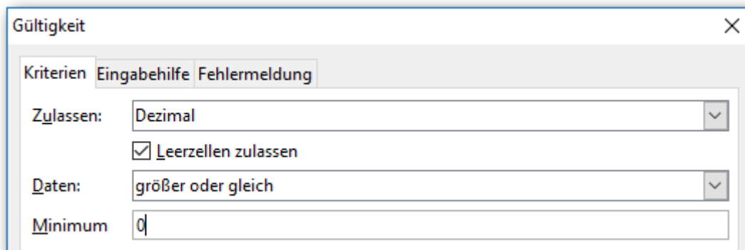
Abbildung 7: Gültigkeit – Kriterien
